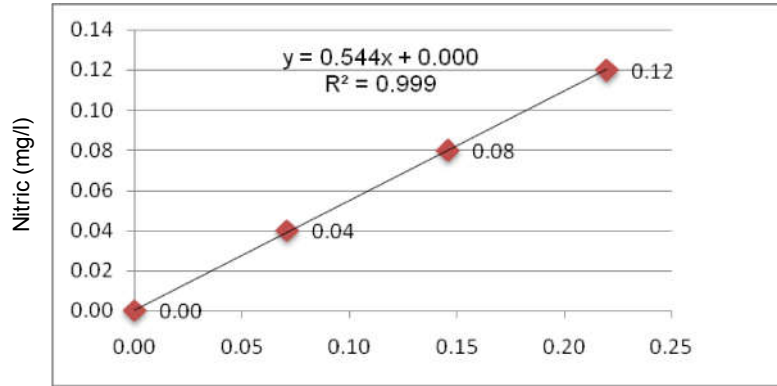
Hình: Đường chuẩn nitrite để xác định hàm lượng nitrate
